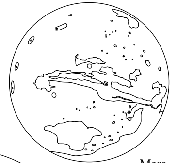
Mars
