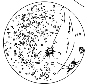
Merkury
