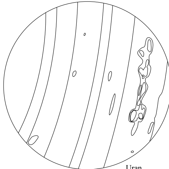
Uran
